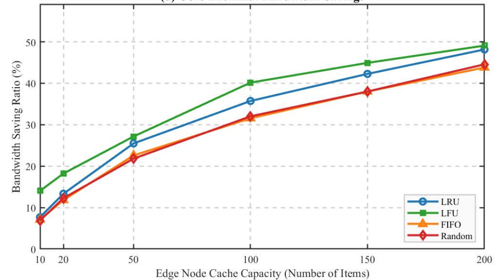
(d) Core Backhaul Bandwidth Savings
